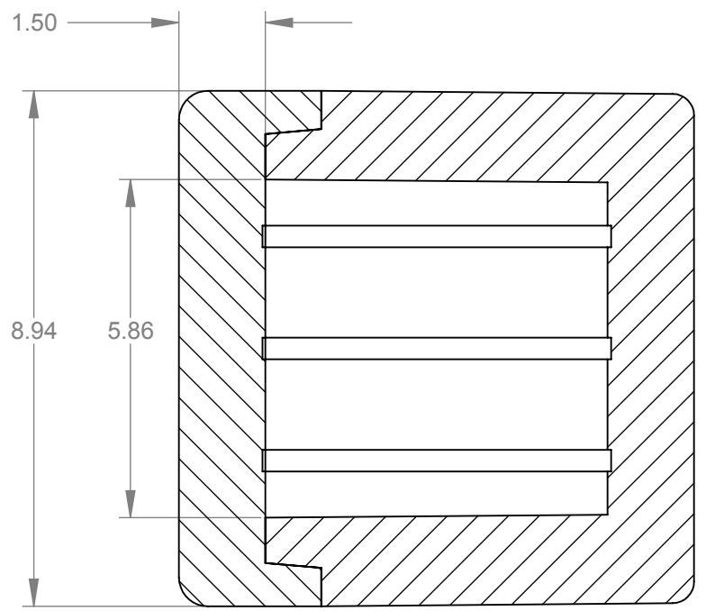
SECTION D-D
